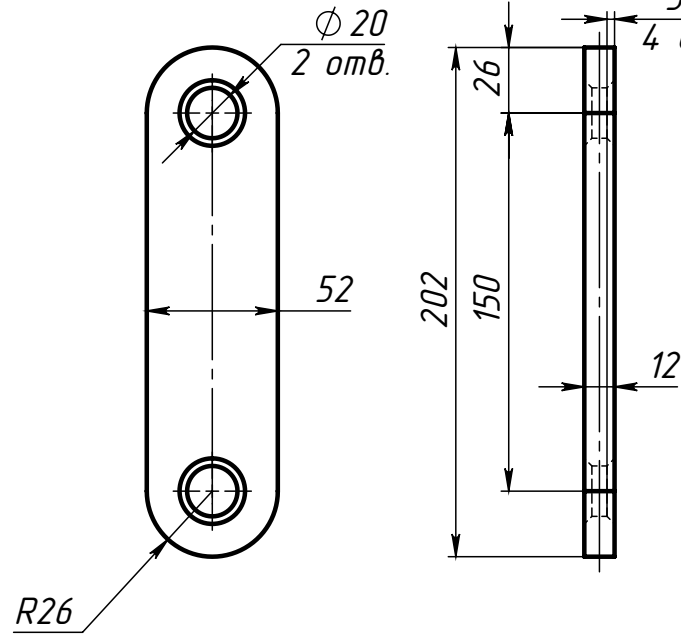
Поз.4 (Серьга 20)
